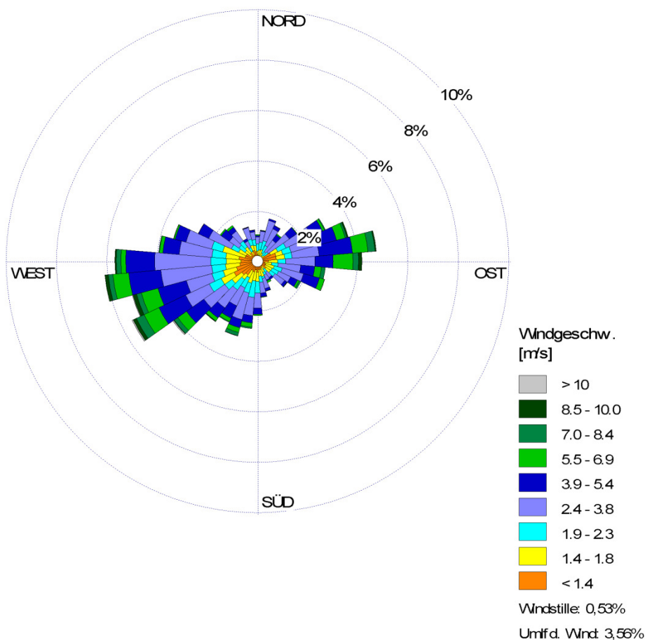
Abbildung 6-2: Windrichtungshäufigkeitsverteilung der Station Celle
