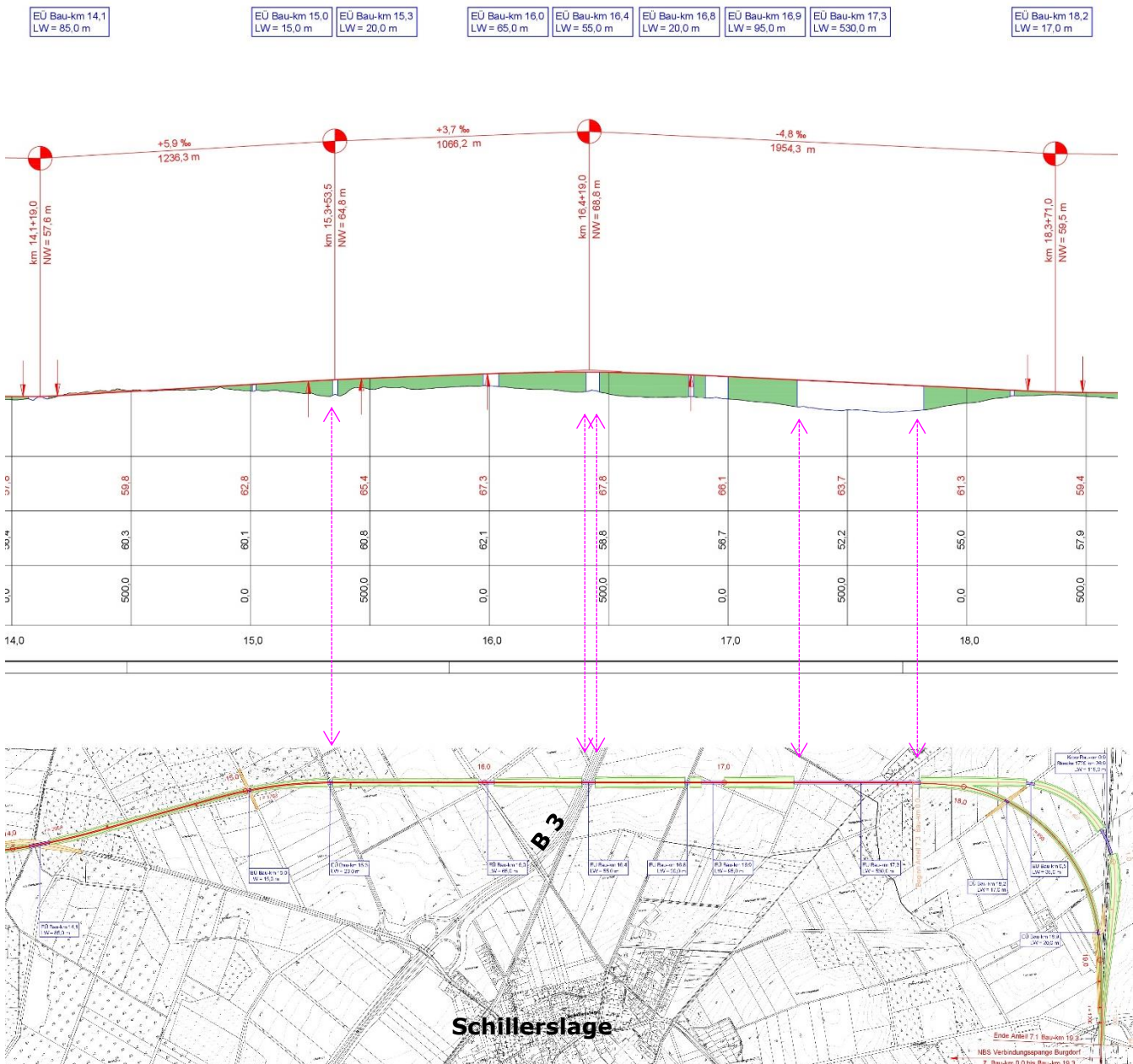
Lageplan, Ausschnitt, ohne Maßstab
