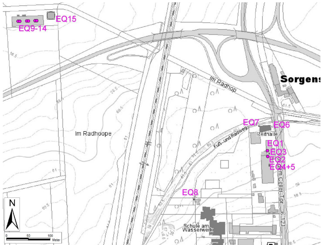
Abbildung 1: Lage der Emissionsquellen IST-Zustand
