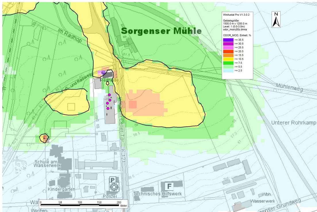
Abbildung 7: Variante 3 - Geruchswahrnehmungshäufigkeiten in [%] der Jahresstunden mit markierter 10 %-Isolinie
