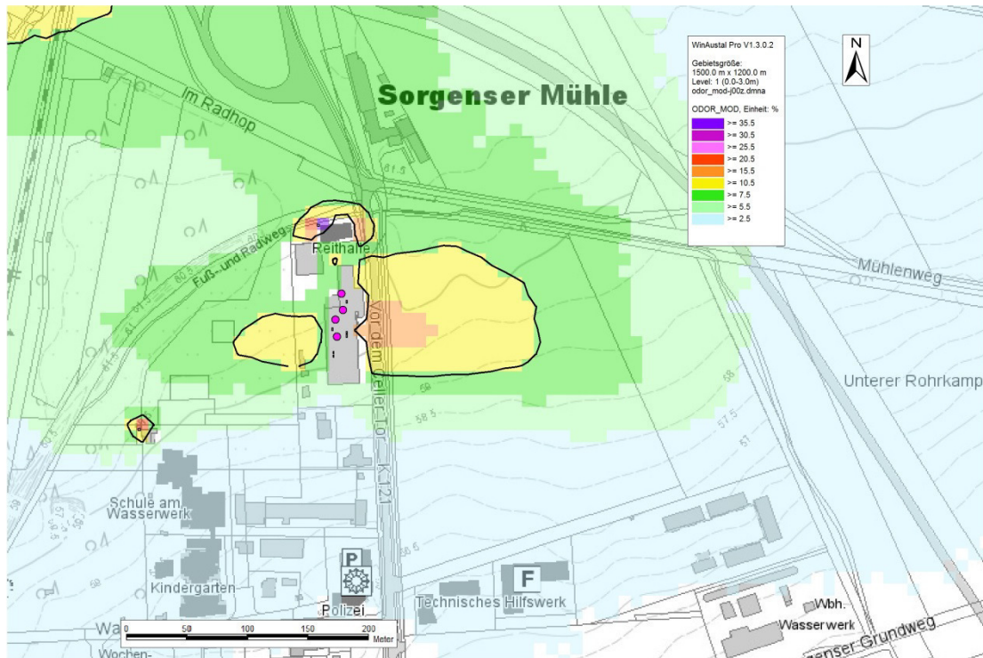
Abbildung 9: Variante 4 - Geruchswahrnehmungshäufigkeiten in [%] der Jahresstunden mit markierter 10 %-Isolinie
