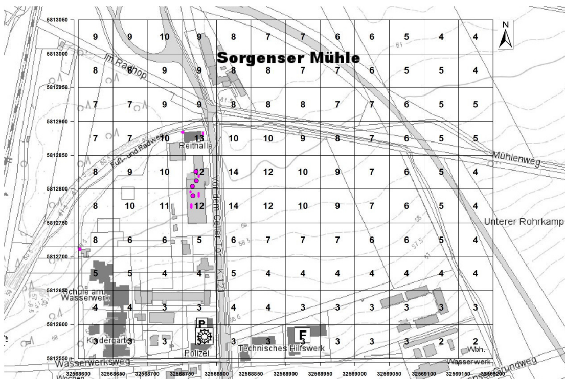
Abbildung 10: Variante 4 - Geruchswahrnehmungshäufigkeiten in [%] der Jahresstunden ausgewiesen für Beurteilungsflächen mit Abmessungen von 50 m x 50 m
