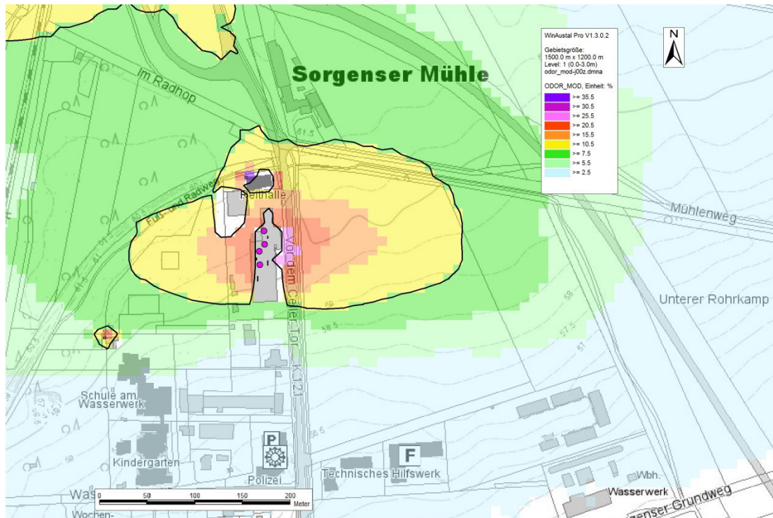
Abbildung 5: Variante 2 - Geruchswahrnehmungshäufigkeiten in [%] der Jahresstunden mit markierter 10 %-Isolinie
