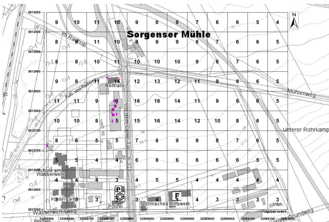
Abbildung 8: Variante 3 - Geruchswahrnehmungshäufigkeiten in [%] der Jahresstunden ausgewiesen für Beurteilungsflächen mit Abmessungen von 50 m x 50 m
