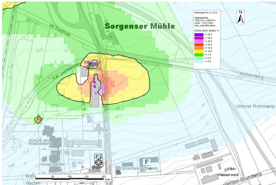
Abbildung 3: Variante 1 - Geruchswahrnehmungshäufigkeiten in [%] der Jahresstunden mit markierter 10 %-Isolinie
