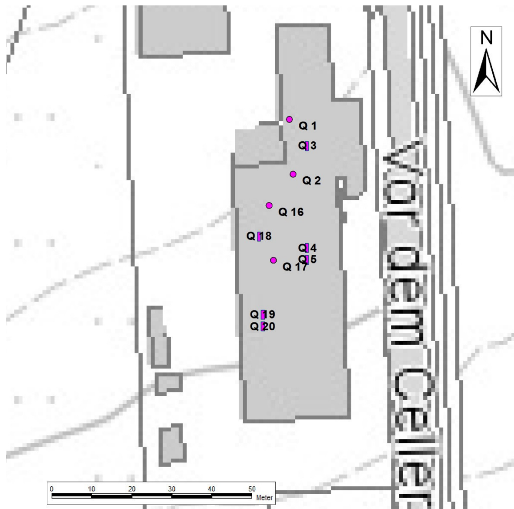
Abbildung 2: Lage der Emissionsquellen PLAN-Zustand (nur Keksfabrik)
